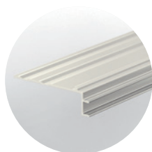
Profilé Incizo / Profilé de base en aluminium Incizo pour escaliers QSINCP(-) / NEINCPBASE(-) 2 150 x 48 x 13 mm / 2 150 x 71 x 20 mm
